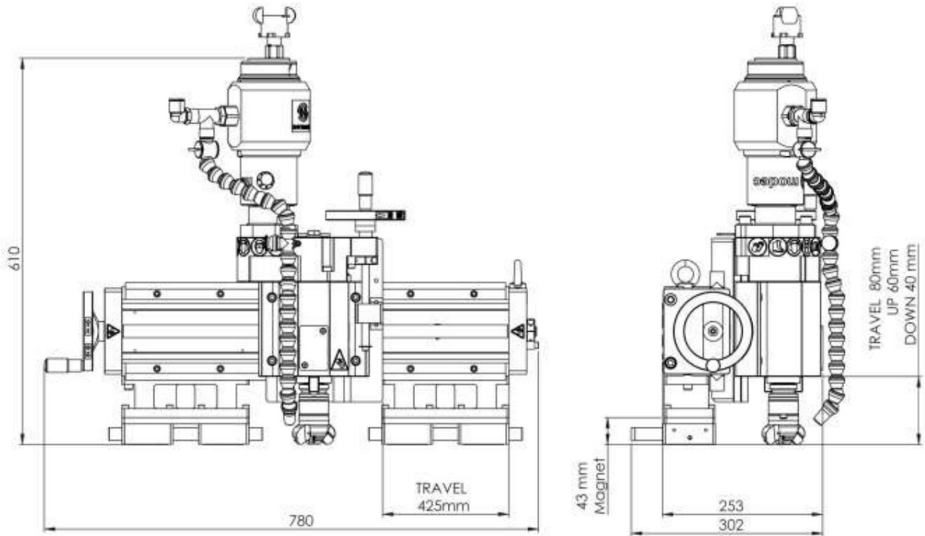
手動送りの機械寸法
