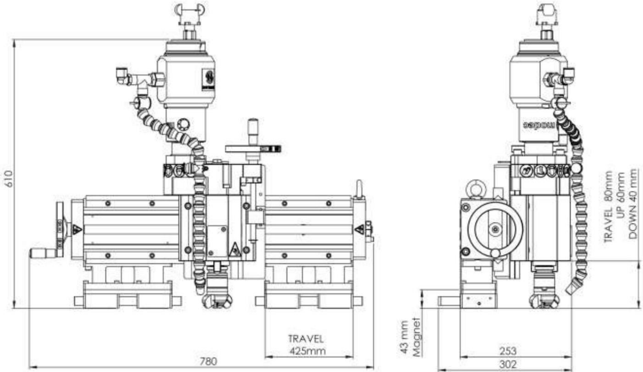
Dimensiones de la máquina con alimentación manual.
